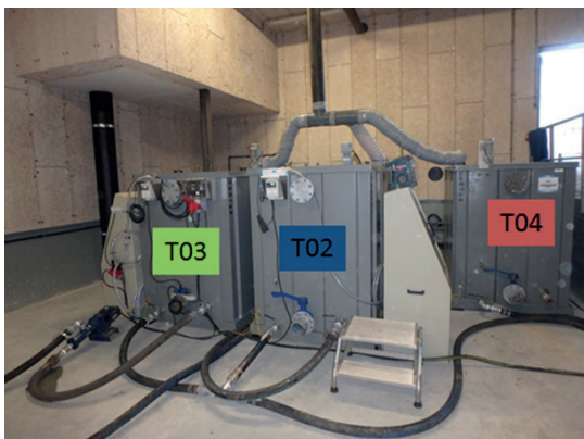
AFBEELDING 2.2 PILOTOPSTELLING KAUMERA-EXTRACTIE OP RWZI APELDOORN
