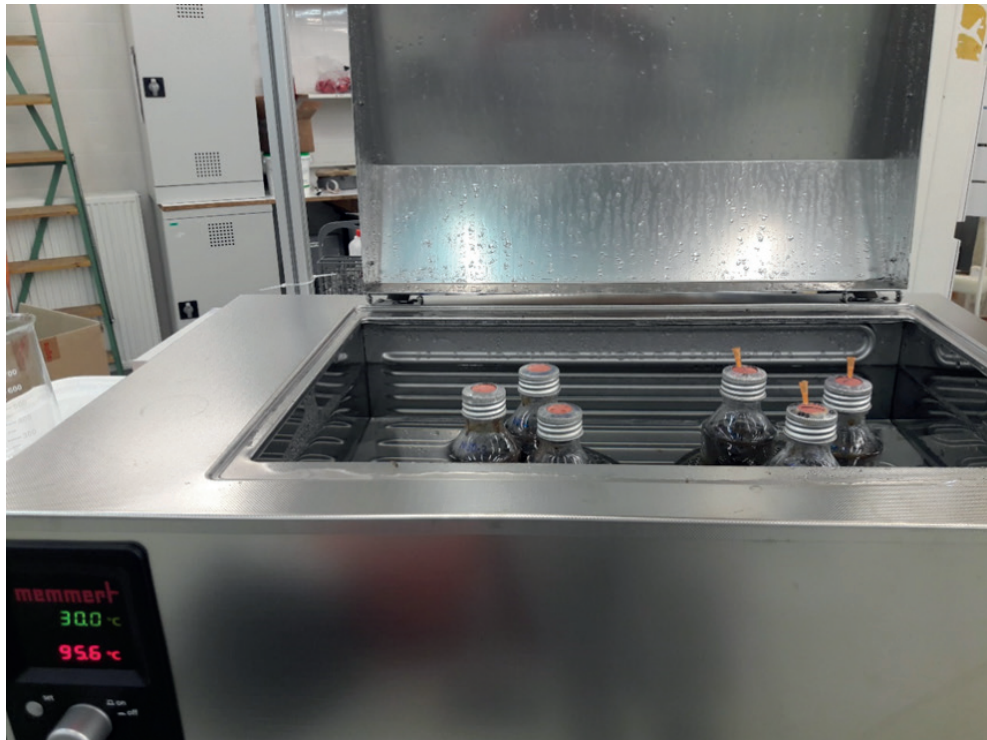
FIGUUR 3.3 OPSLAG VAN GEËXTRAHEERDE KAUMERA BIJ 30 C. LINKS: AFGESLOTEN FLESJES ZONDER ZUURSTOF (HEADSPACE GEFLUSHT MET STIKSTOFGAS, RECHTS: OPEN VERBINDING MET DE LUCHT VIA EEN NAALDJE DOOR HET SEPTUM)
