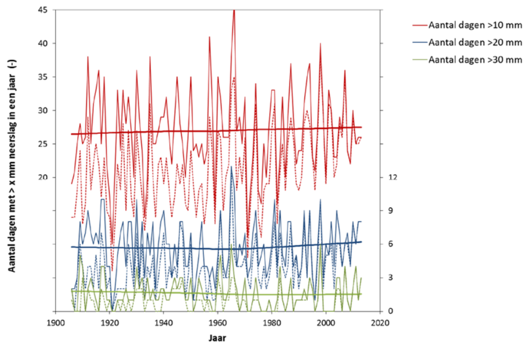
FIGUUR 4.5 HET AANTAL DAGEN MET Overschrijding VAN EEN NEERSLAGSM IN DE BILT VOOR DE PERIODE 1906-2014. GESTIPPELDE LIJN VOOR DE GEHOMOGENISEERDE REEKS EN DOORGETROKKEN LIJN VOOR DE BASISREEKS 2014. HET AANTAL DAGEN >10 MM STAAT OP DE LINKER Y-AS, HET AANTAL DAGEN >20 EN >30 MM OP DE RECHTER Y-AS. DE GLADDE CURVES ZIJN HET RESULTAAT VAN EEN LOESS FIT (DEGREE =1, FAMILY=GAUSSIAN, SPAN=0.9)
