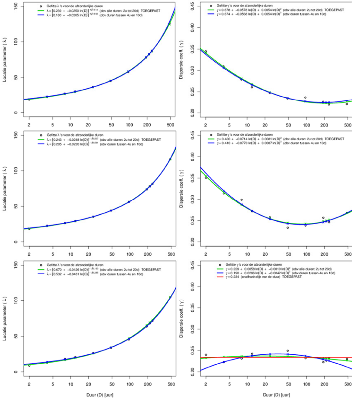
FIGUUR 2.2 LOCATIE-DUUR (LINKS) EN DISPERSIE-DUUR (RECHTS) RELATIES VOOR NEERSLAGDUREN TUSSEN 2 UUR EN 20 DAGEN OP JAARBASIS (BOVEN), VOOR MAART T/M OKTOBER (MIDDEN) EN VOOR NOVEMBER T/M FEBRUARI (ONDER) VOOR DE BILT. RONDJES ZIJN DE INDIVIDUEEL PER DUUR GEFITTE WAARDEN
